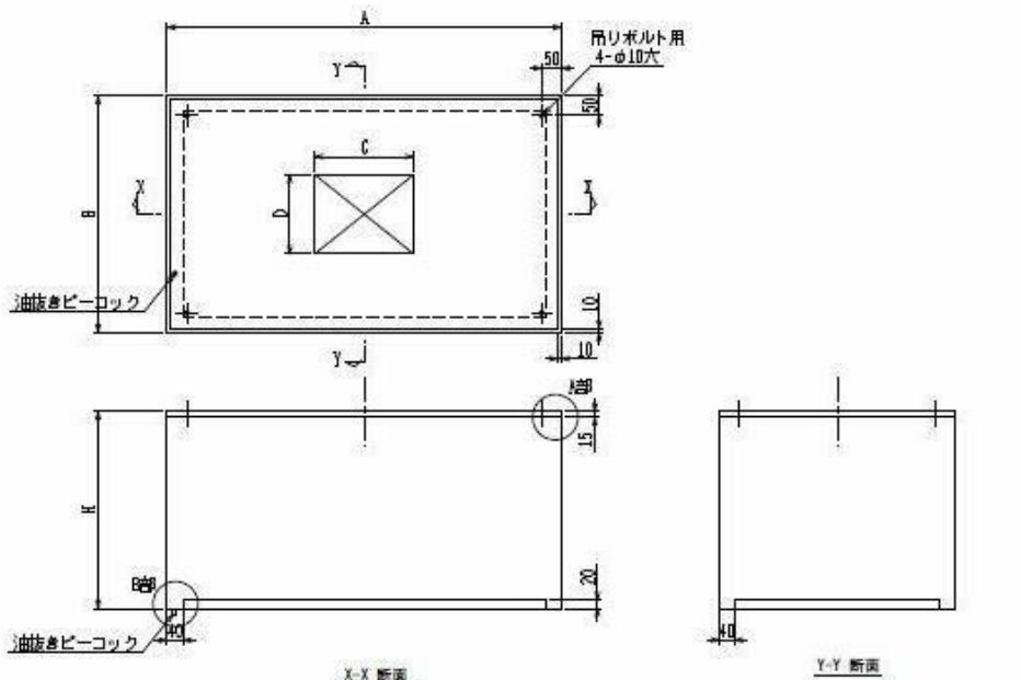
X-X 断面
